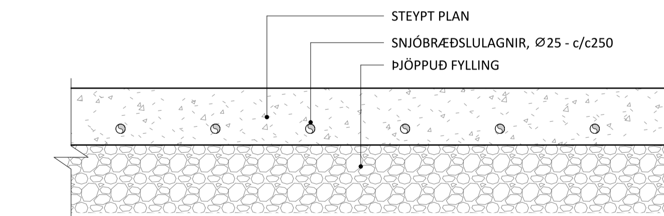
KENNISNIÐ SNJÓBRÆDSLULA STEYPA 1 : 10
