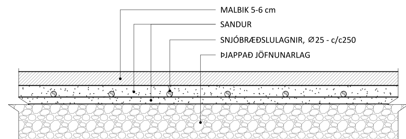
KENNISNIÐ SNJÓBRÆDSLULA MALBIK 1 : 10
